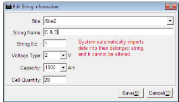
Рис. 4.2.2.г Для цепочки элементов (String)
